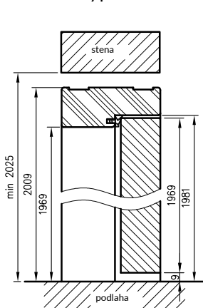
Zvislý prierez OPB
