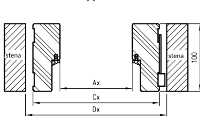
pre bezpodrážkové dvere jednokridlové
