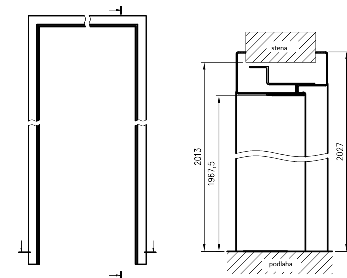
Variety zárubní vzhľadom na hrúbku steny
