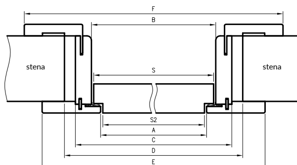
D - požadovaná šírka otvoru v múre
