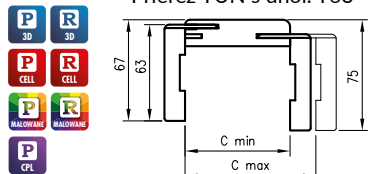
Prierez TUN s uhol. T63
