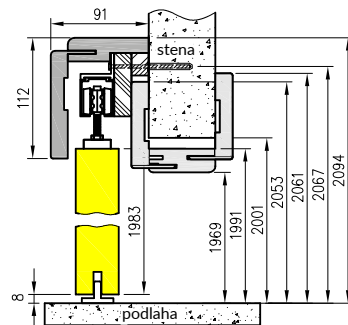
Výška krídla bez poldrážky - 1983 mm
