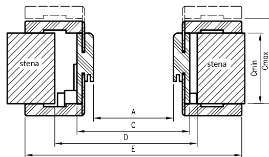
Pozdĺžny prierez ORB
