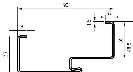
Profil zárubne:
