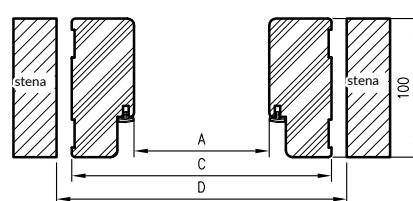
pre poldrážkové dvere jednokridlové
