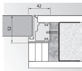
Bezpolodrážkové (otvorenie smerom von)
