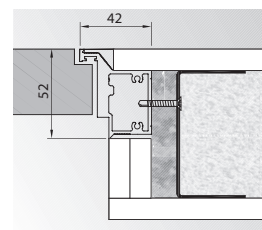
Opačná polodrážka (otvára sa dovnútra)
