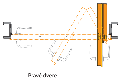
SPÔSOB OTVÁRANIA DVERÍ (pohľad zhora)
