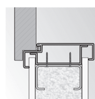
zárubňa rohová VELKÁ montáž na SDK stenu
